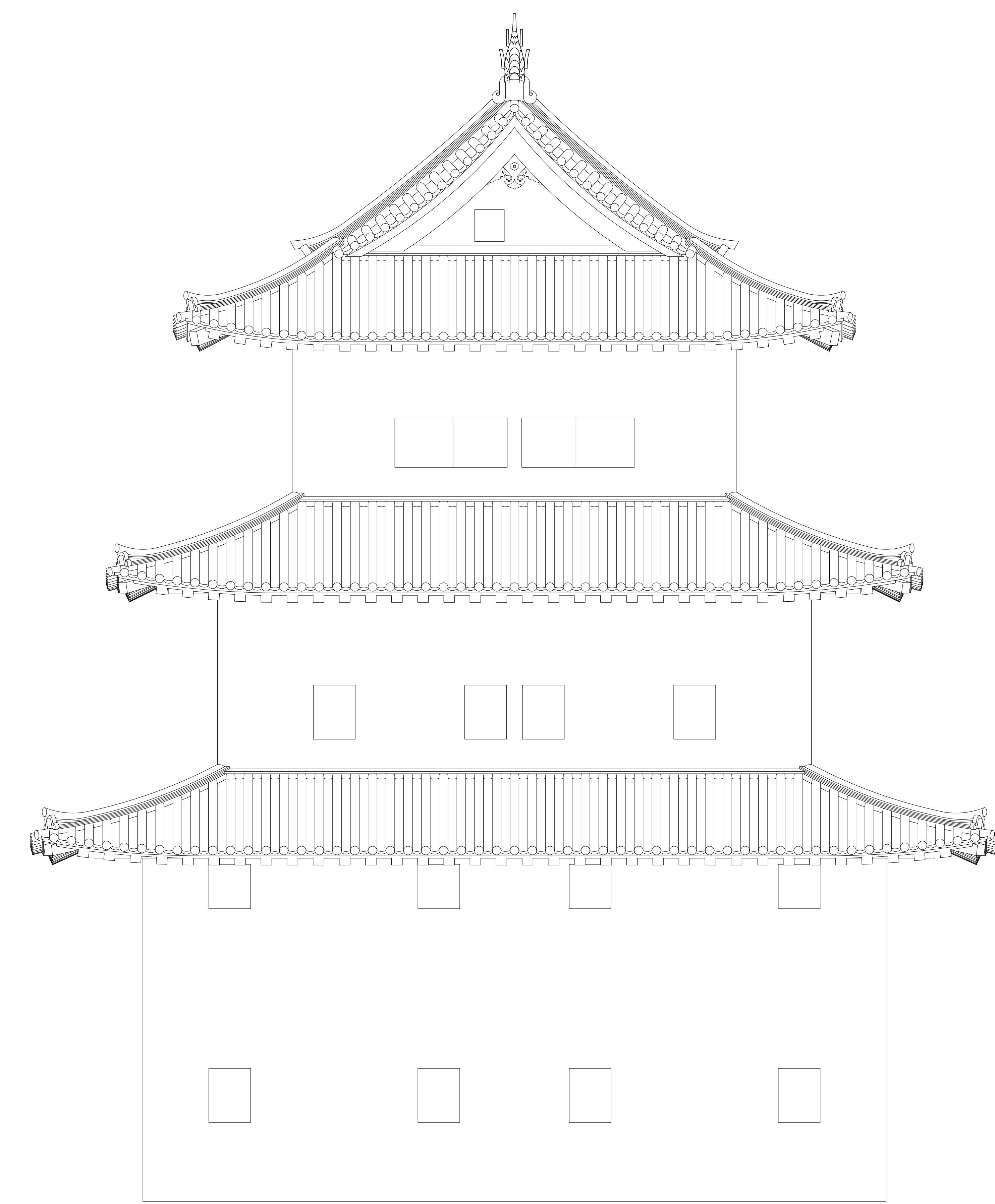
北面
