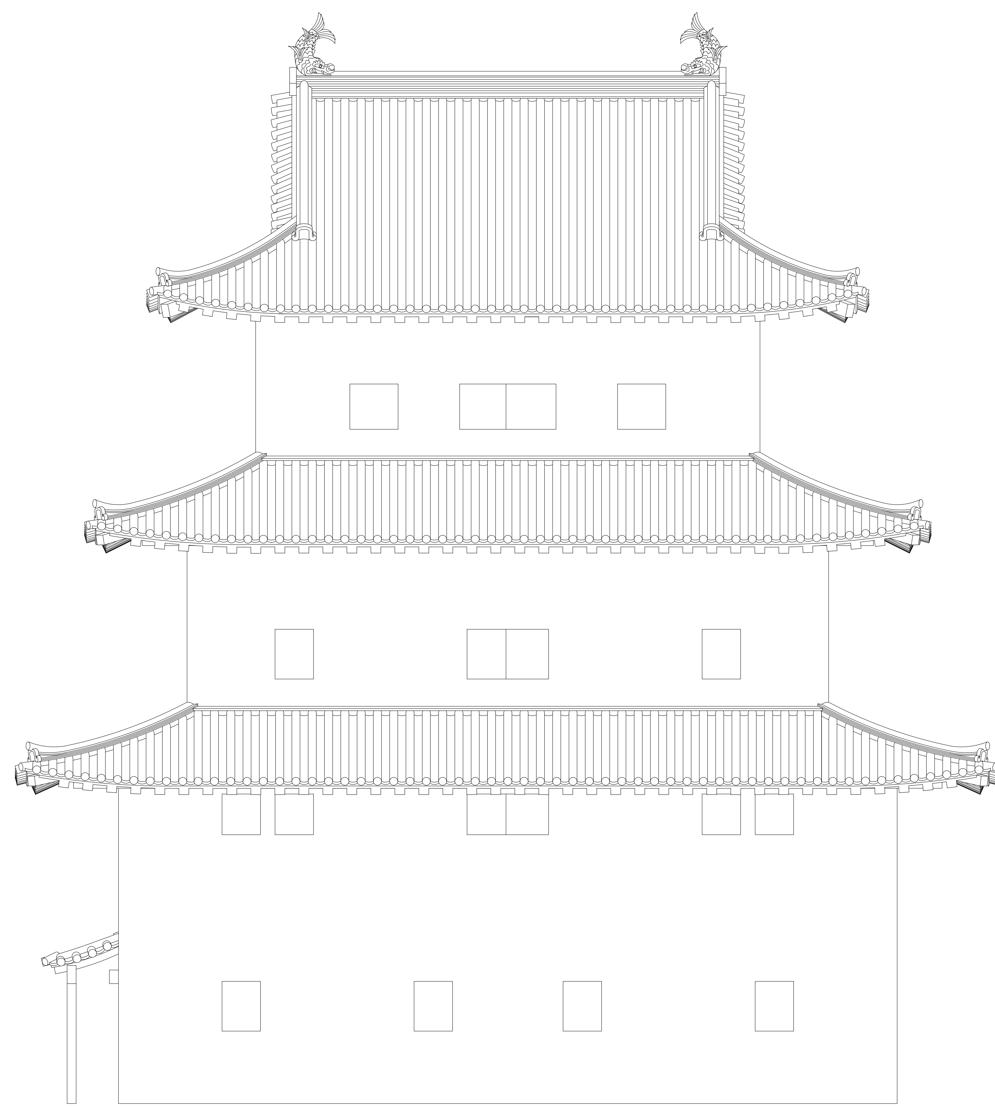
東面
